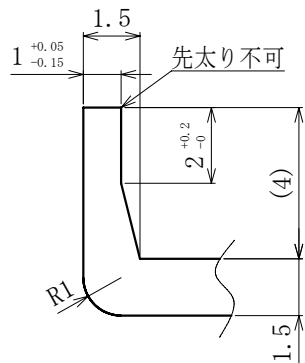
2-A部詳細(5/1)
