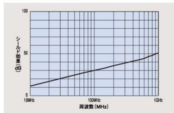
●周波数とシールド効果 (磁界)
