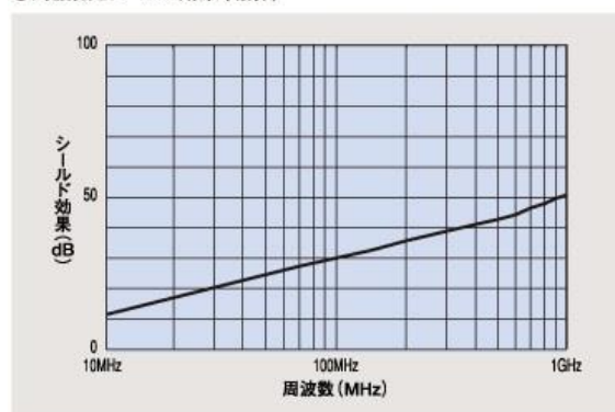
●周波数とシールド効果 (磁界)
