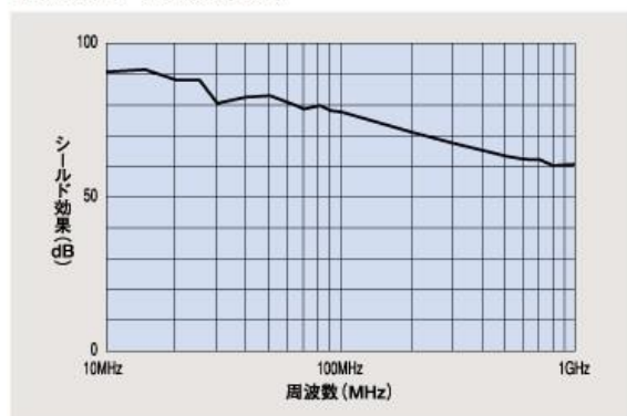
●周波数とシールド効果 (電界)
